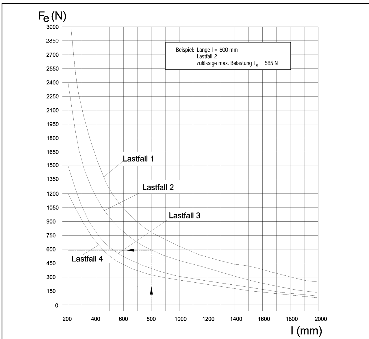
Lastfall 1
